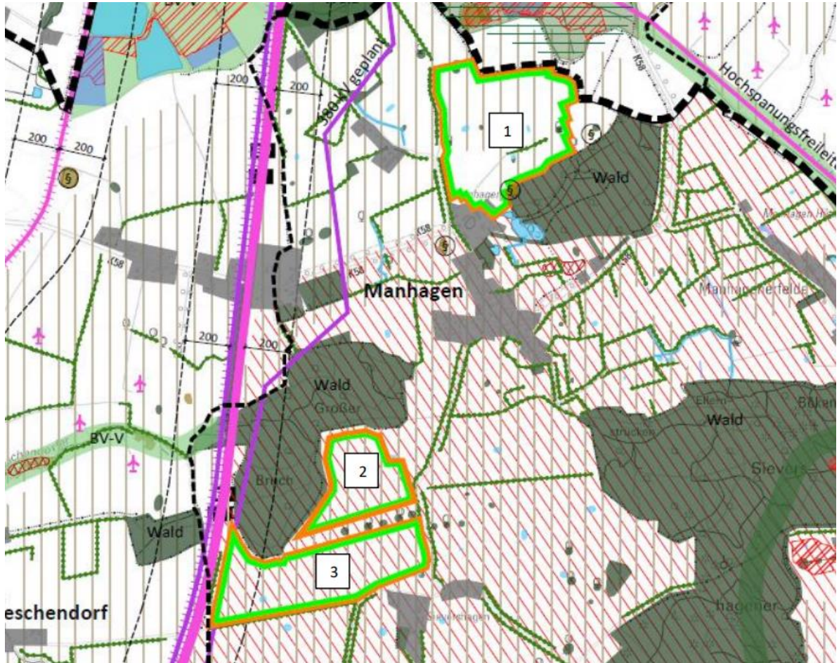
Abb.: Standortkonzept Manhagen für Freiflächen-Photovoltaikanlagen mit Nummerierung der Teilflächen, Quelle: ELBBERG, Hamburg, 04.03.2022
